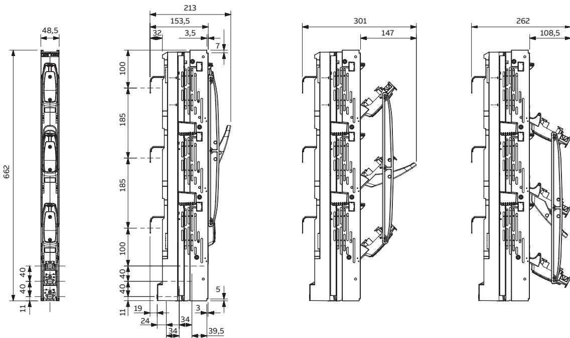
ZHBM00-3P
