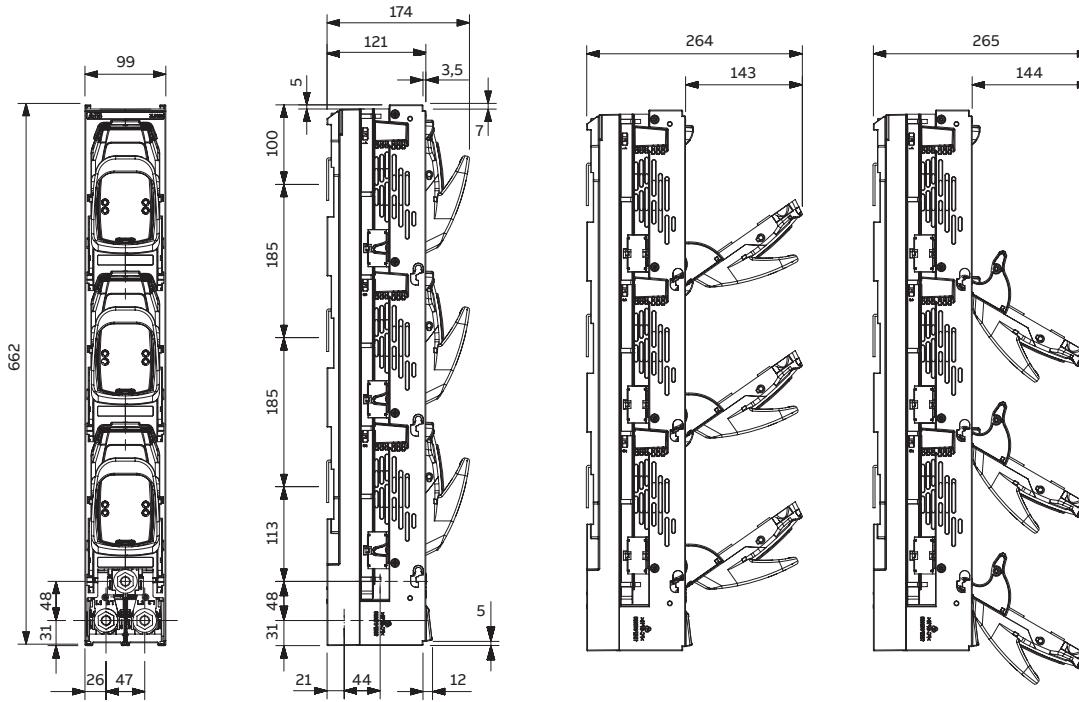
ZLBM1/2/3 -1P
